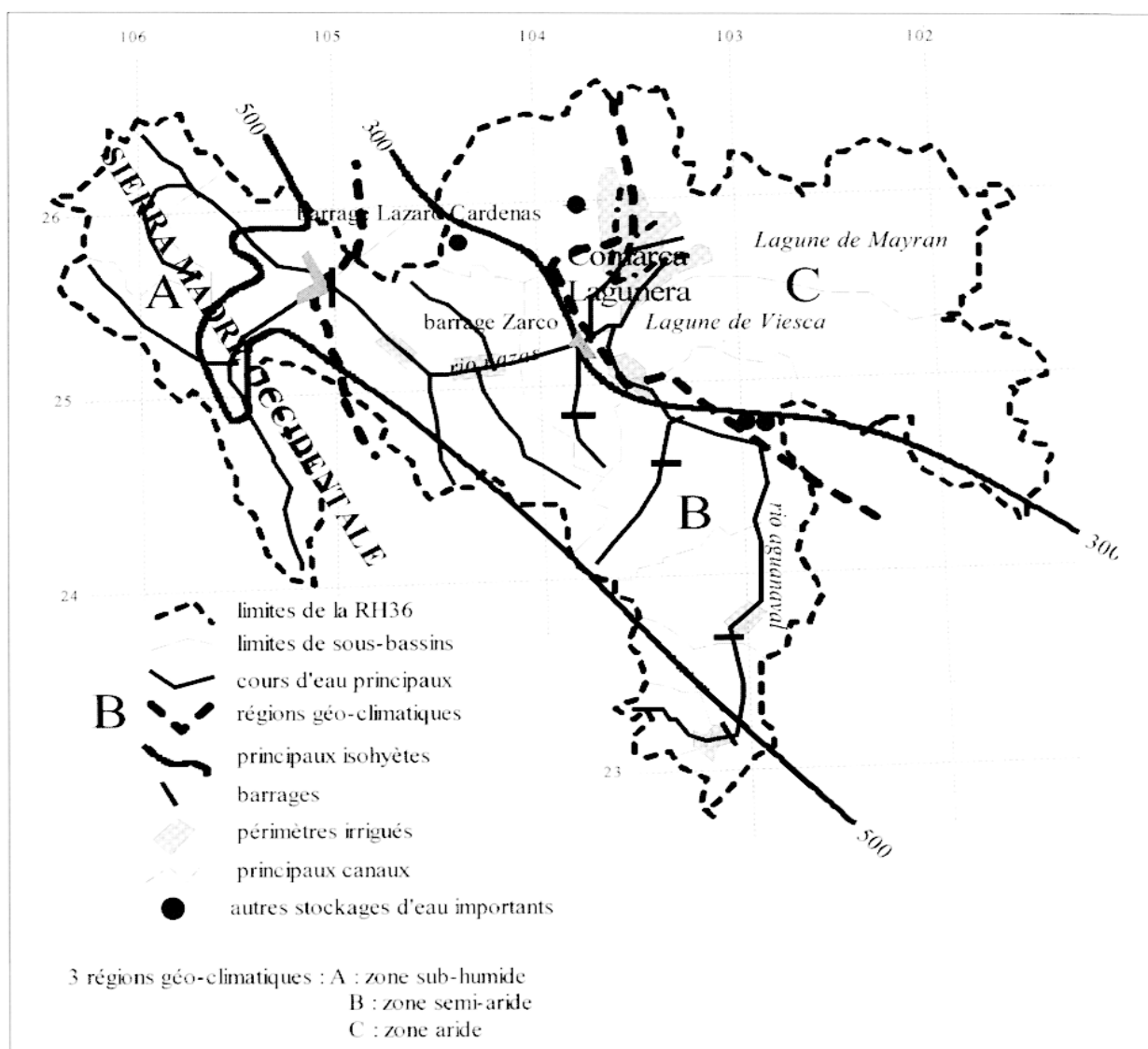
Figure 5 : Les 3 zones géoclimatiques de la RH 36
