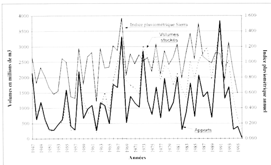
Figure 8 : Retenue El Palmito. Apports et volume stockés. Indice pluviométrique annuel de la Sierra Madre occidentale
