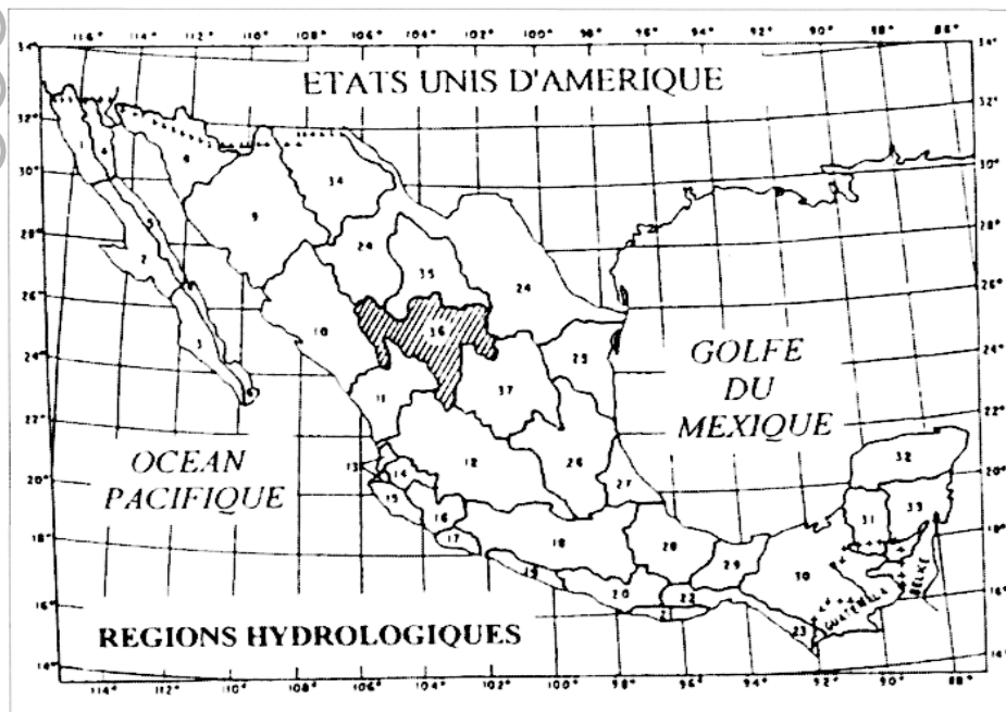
Figure 1 : Localisation de la RH 36, bassin versant des rios Nazas et Aguanaval
