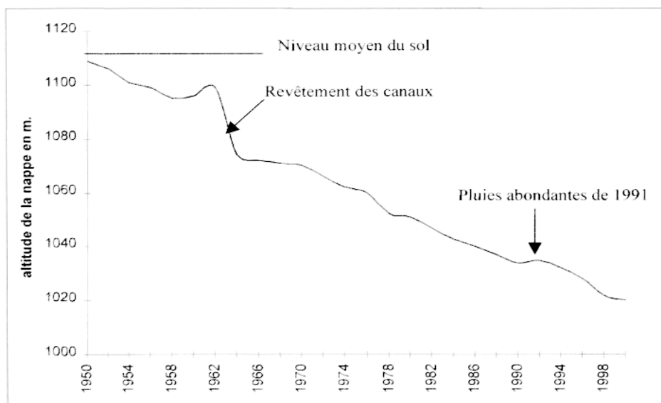
Figure 6 : Abaissement du niveau phréatique depuis 1950 dans la Laguna
