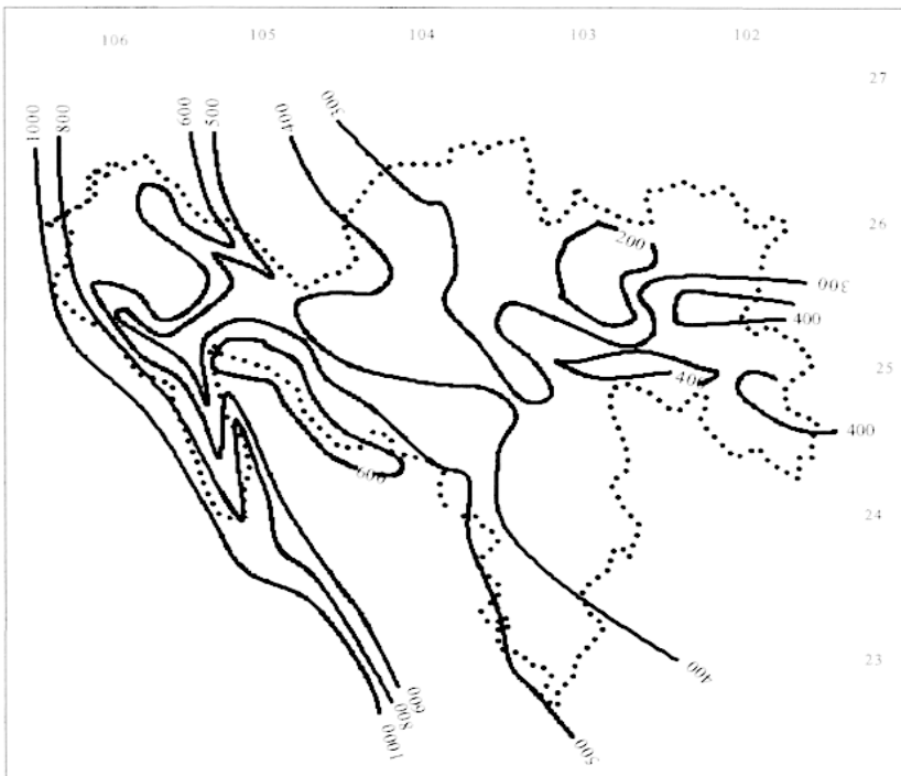
Figure 2 : Isohyètes annuelles moyennes dans la région hydrologique n° 36
