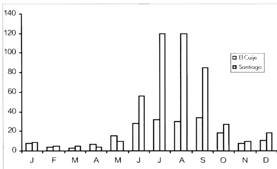
Figure 3 : Pluviométrie annuelle à Santiago Papasquiari et EL Cuije
