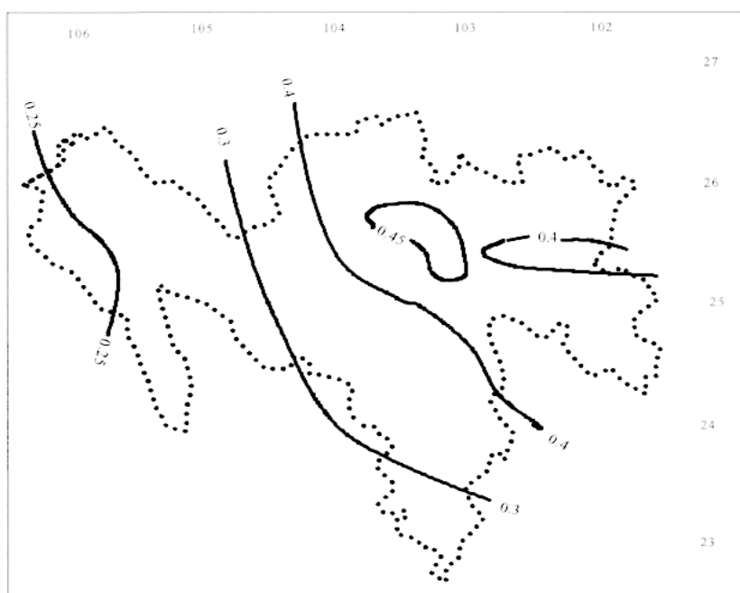
Figure 4 : Coefficient de variation des précipitations annuelles dans la RH 36
